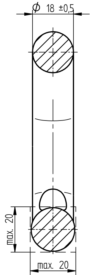
Schnitt A-A
